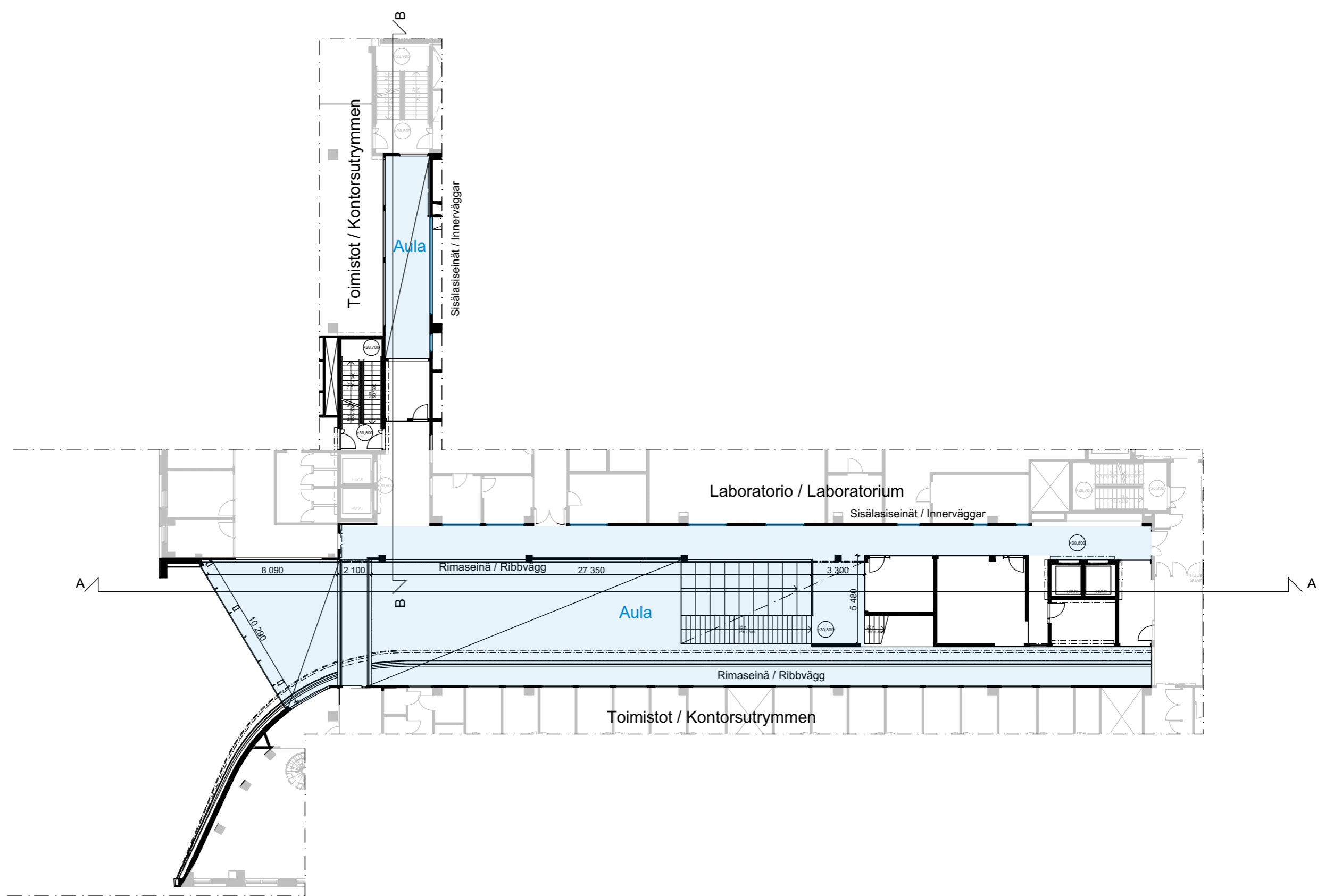
3. kerros / 3. våningen - pohjapiirros / plan 1:250
