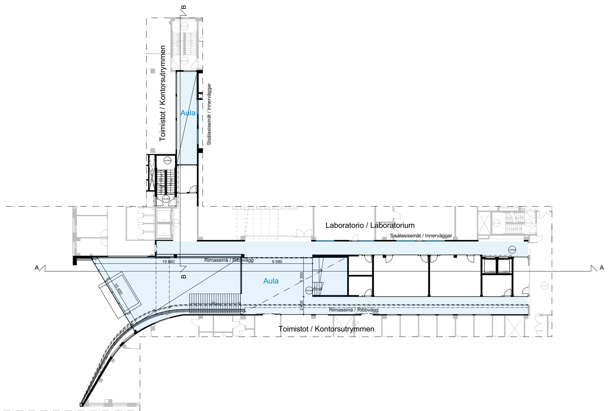
2. kerros / 2. våningen - pohjapiirros / plan 1:250
